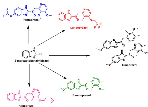
Figura 6. Compuestos orgánicos derivados del 2-mercaptobenzimidazol evaluados en el acero API 5L X52
