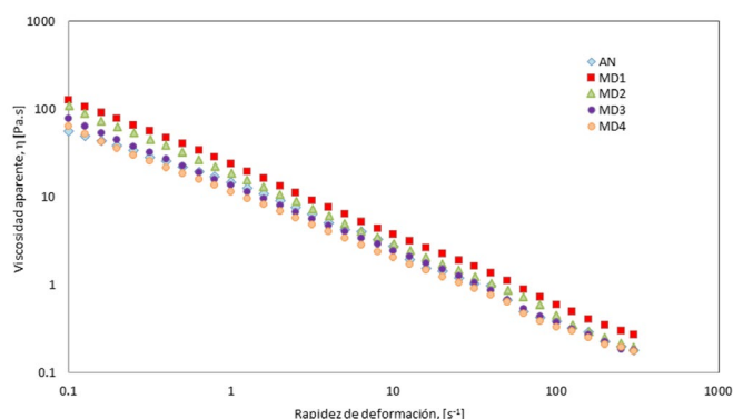
Figura 6. Curvas de flujo de almidones modificados dualmente ensayados a 4 niveles de concentración por métodos químicos; AN=almidón nativo; MD1=Almidón dualmente modificado 1; MD2=Almidón dualmente modificado 2; MD3=Almidón dualmente modificado 3 y MD4=Almidón dualmente modificado 4
