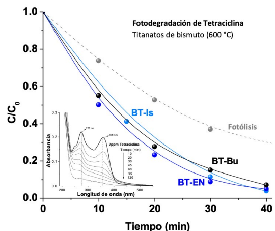
Figura 3. Concentración relativa de la fotodegradación de tetraciclina, usando titanatos de bismuto en radiación UV. Espectro de absorción de tetraciclina (Insertada)
