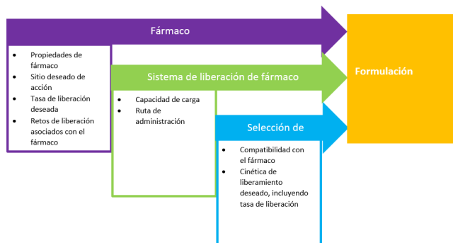
Figura 3.- Proceso de selección en la formulación en sistema de liberación de fármacos
