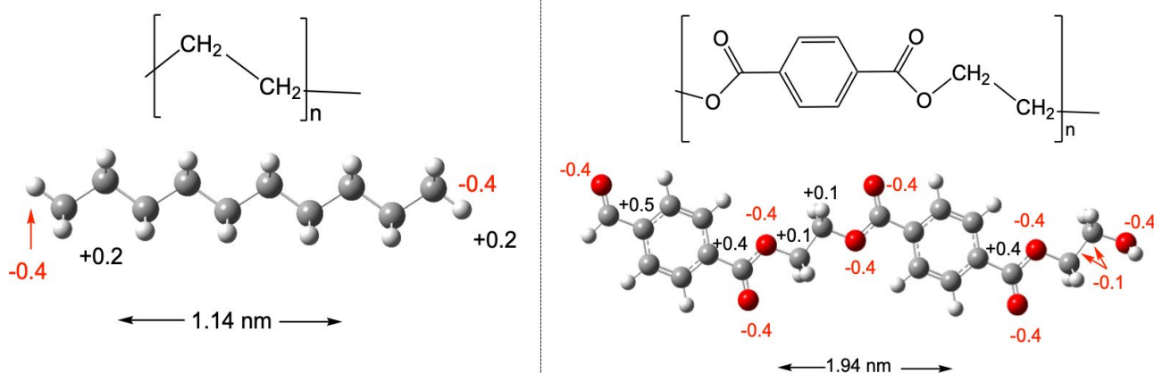
Estructuras optimizadas de los dos modelos. Se incluyen los valores de la longitud de la molécula y de las cargas atómicas de Mulliken
