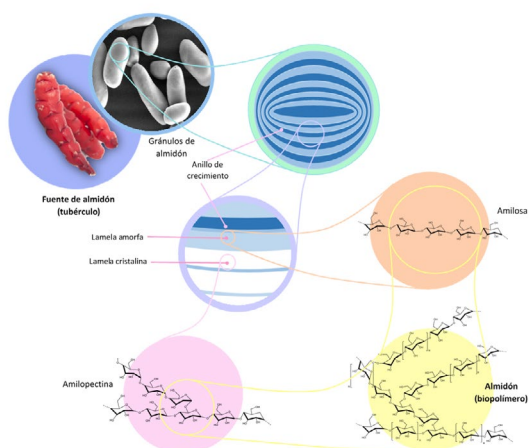
Figura 1. Estructura química del almidón (biopolímero) [modificado de Adewale et al., 2022]
