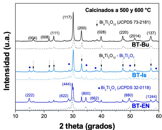
Figura 1. Difractograma de titanatos de bismuto calcinados a 500 y 600 °C, preparados en diferentes solventes
